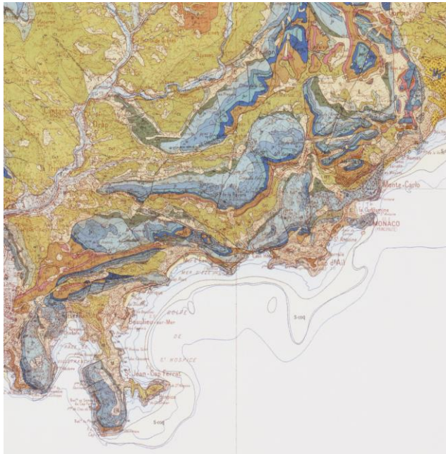
Extrait de la carte géologique au 1/50000 Menton-Nice
